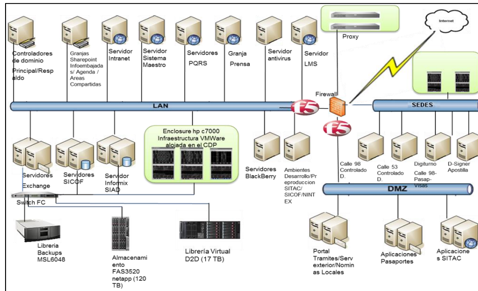
Ilustración 3 Arquitectura general de los servicios tecnológicos FUENTE: Dirección de Gestión de Información y Tecnología
